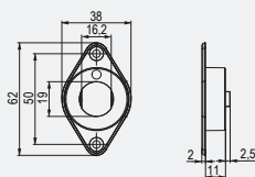
309274 adaptér na montáž do dreva
