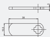
309275 závora 310 rovná
