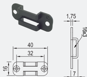
Vodidlo tyče
