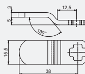
309276 závora 390 zakrivená
