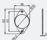
350805 plastová vložka pre montáž do tenkého dreva, nutné kombinovať s adaptérom 309274
