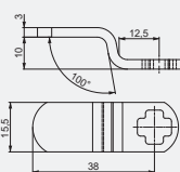
309277 závora 400 zakrivená
