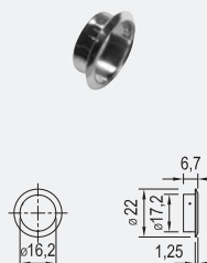
Rozeta 16,5 mm
