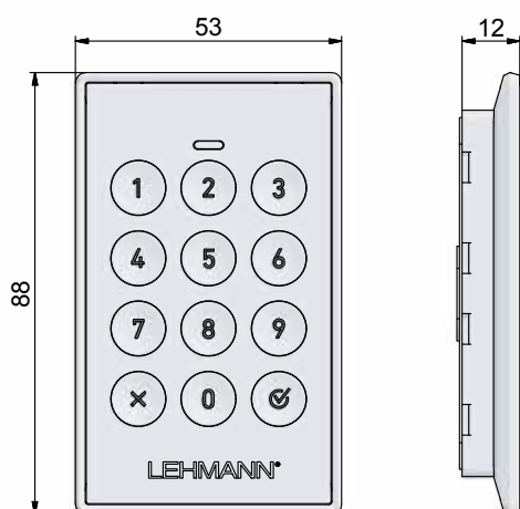
Keypad without labelling clip Klávesnice bez popisovacího klipu
