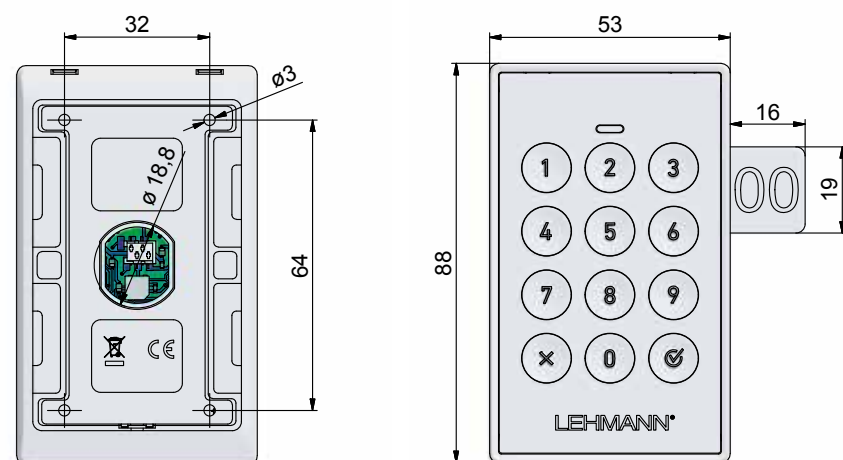
Keypad with labelling clip Klávesnice s popisovacím klipem
