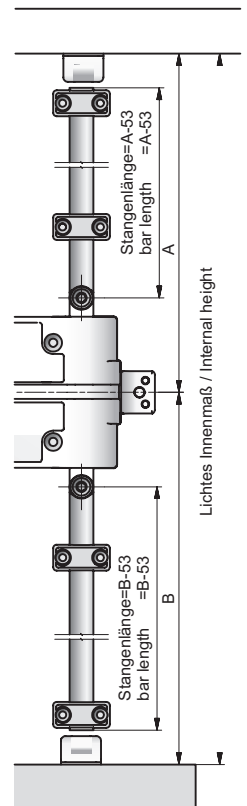
Installation dimensions Stangenlängenberechnung
