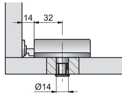
Shown in locked position Darstellung geschlossen
