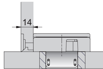
Shown in locked position Darstellung geschlossen
