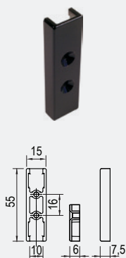
Zaczep blokujący
