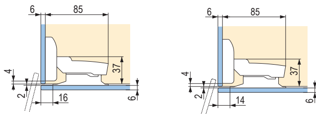
Úplne naložené dvre (bez medzery)
