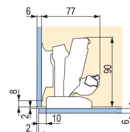
Naložené dvre s medzerou 2 mm
