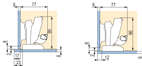
Naložené dvre s presahom dverí 11 mm
