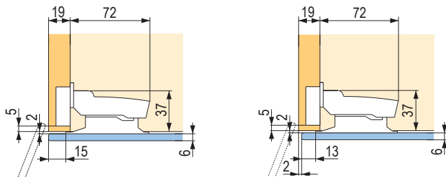
Úplne naložené dvre (bez medzery)
