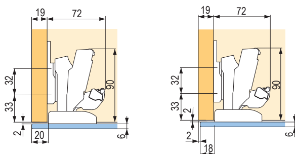
Naložené dvre s medzerou 2 mm
