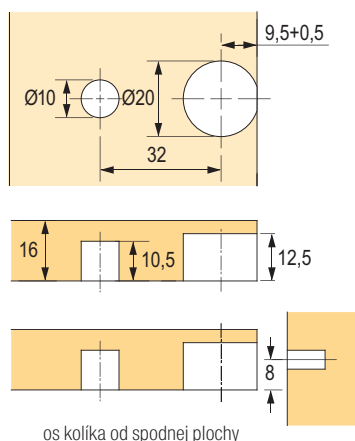
schéma vŕtania dielca
