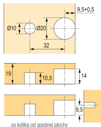
schéma vŕtania dielca
