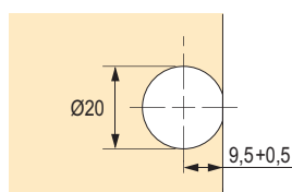
schéma vŕtania dielca
