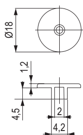
krytka excentra
