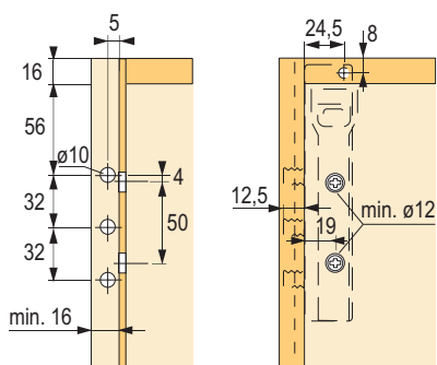
závesné kovanie SAH 216
