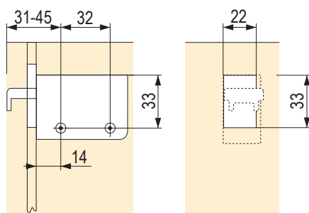
Upevňovacia pozícia v bloku korpusu a vo výreze v zadnej stene
