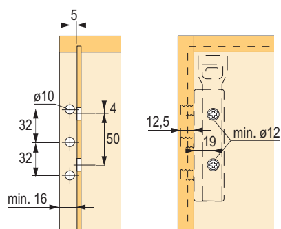
závesné kovanie SAH 215
