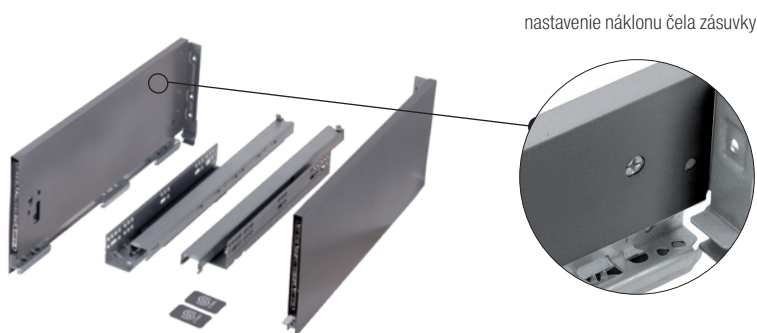
nastavenie náklonu čela zásuvky
