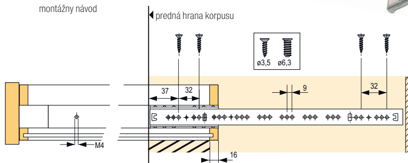
montážny návod
