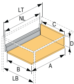
Čelná zásuvka, výška 70/176 mm
