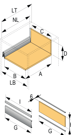
Vnúťorná zásuvka, výška 94 a 126/218 mm
