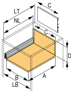
Vnúťorná zásuvka, výška 94 a 126/282 mm
